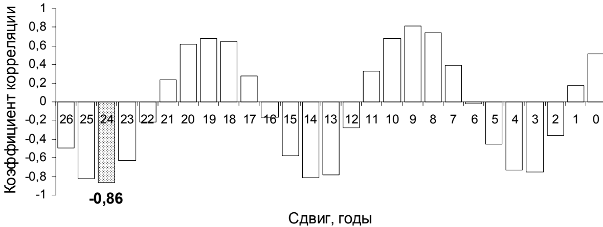
Рис. 2. Коэффициенты корреляции солнечной активности и динамики численности москочки при последовательном сдвиге с шагом 1 год. Выделено максимальное значение.
