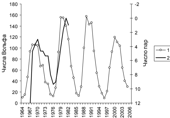
Рисунок 3. Динамика численности москочки (2) и солнечная активность (1). Кривая динамики численности перевернута и сдвинута на 24 года назад.
