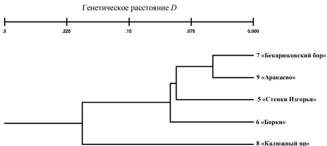
Рис. 3. Дендрограмма генетических расстояний по Неи [16] (UPGMA) между популяциями Ch. tridens
