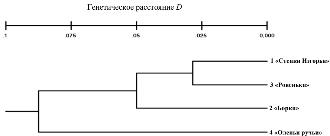
Рис. 2. Дендрограмма генетических расстояний по Неи [16] (UPGMA) между популяциями Br. fruticum
